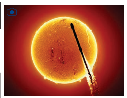
عبور فالکون از مقابل خورشید
